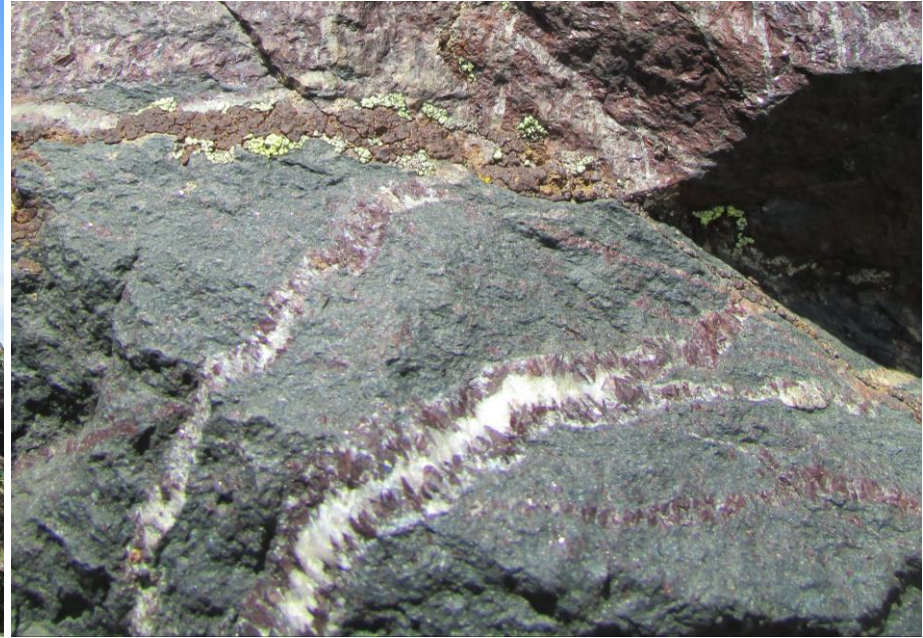
Les veines à magnétite et quartz (quartz en peignes)
